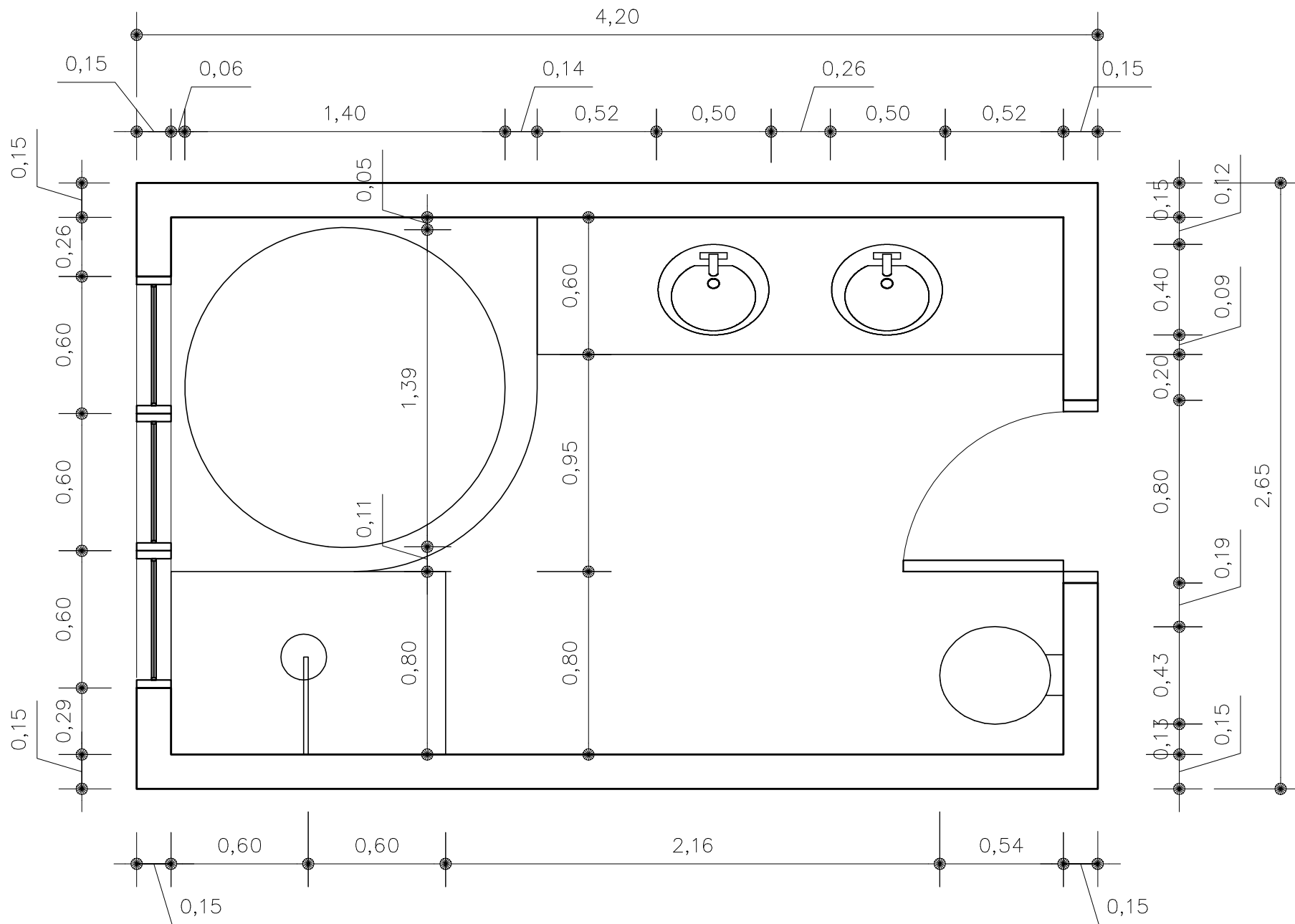
Planta-baixa
